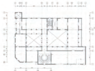
臺南安平案，原 RC 造的結構設計需用 25 公分厚的承重牆，改成 CLT 木構造後，結構計算牆厚只需 14 公分。(圖片來源：rjc 結構公司)
